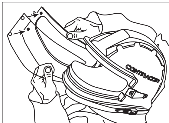
Рис. 3. Замена стёкол шлема Aspect
