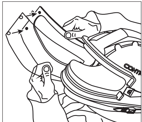
Abb. 3. Austausch der Einwegscheibe(n) Aspect
